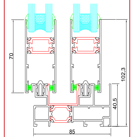
Sección vertical marco cerrado
