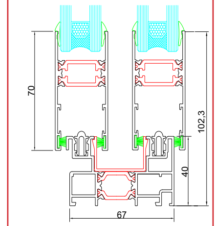
Sección vertical marco abierto
