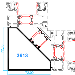
Esquinero de 90°
