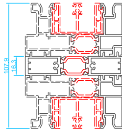
Unión marco con marco corredera
