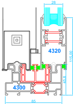
Marco de corredera Hoja de corredera
