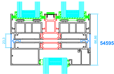
Unión marco corredera con fijo 54595
