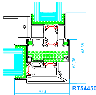
Encuentro en esquina 90° sin parteluces
