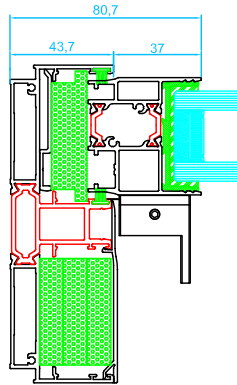
Marco de corredera sección lateral Hoja de corredera
